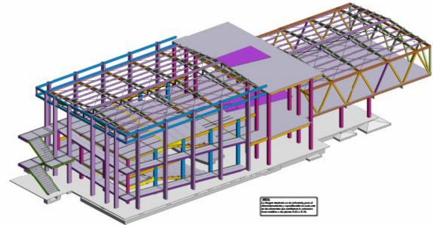
DISEÑO ESTRUCTURAL
